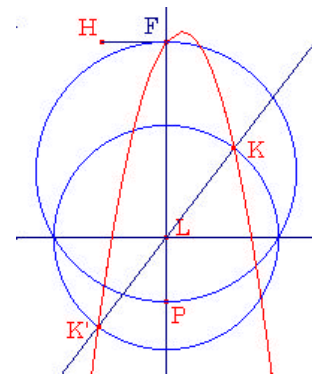
【図】放物線
