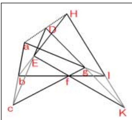
図 14 cbE と gIK の交線は aDH
