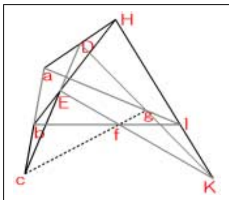
図 1 - 1 DEK と abl が接する場合、cf が交線となる。
