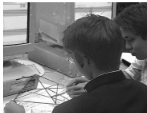
図 15 模型を観察しどこが交線になるか
